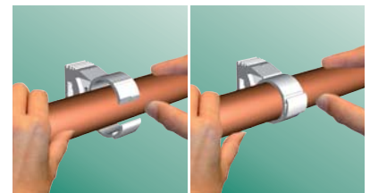
Vložte potrubí do objímky
